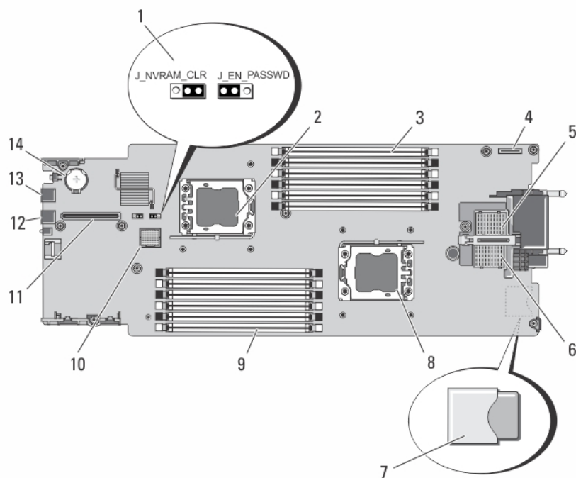
図 21. システム基板のコネクタ
