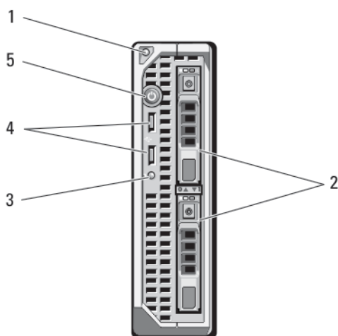
図 1. 前面パネルの機能とインジケータ
