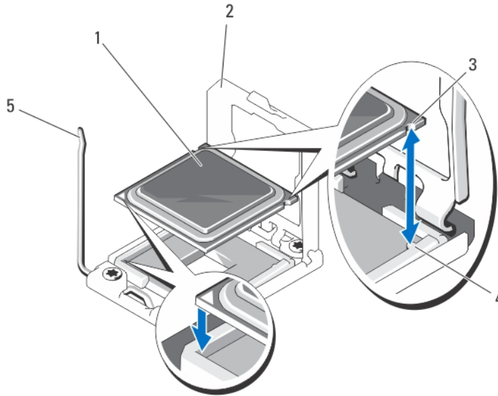
図 14. プロセッサの取り外しと取り付け
