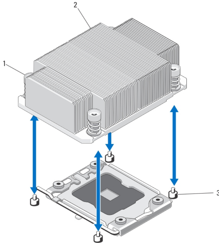
図 13. ヒートシンクの取り外しと取り付け
