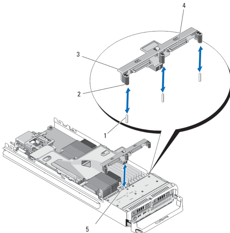
図 17. ハードドライブ /SSD バックプレーンの取り外しと取り付け
