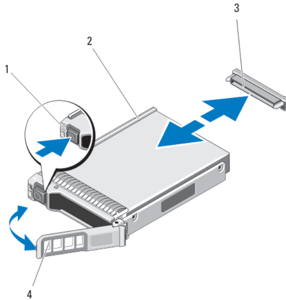
図 15. ハードドライブ /SSD の取り外しと取り付け
