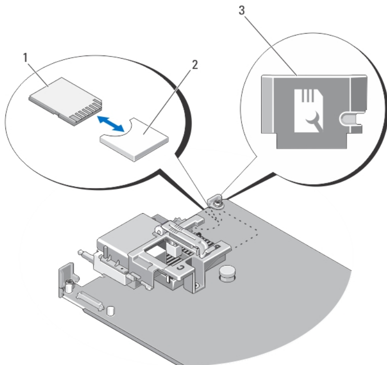
図 12. SD vFlash カードの交換 / 取り付け
