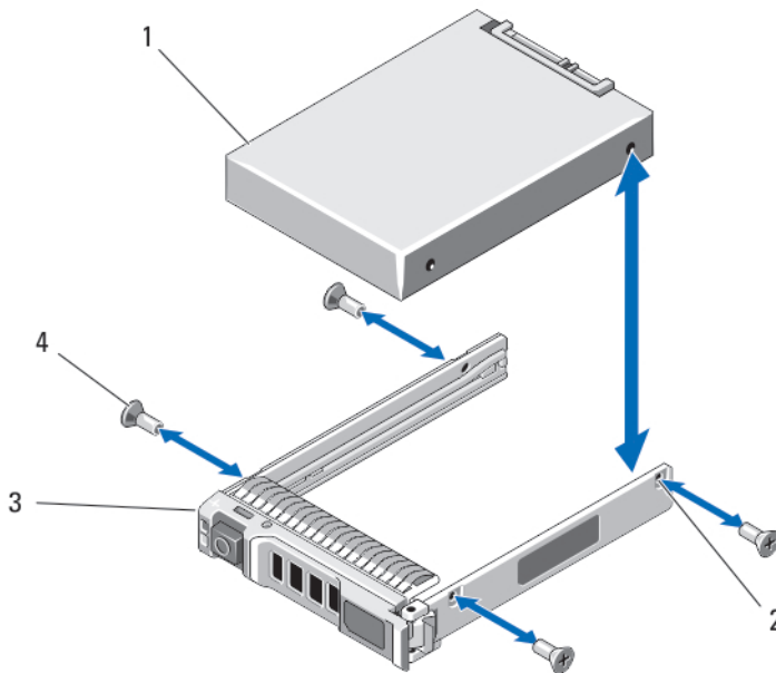
図 16. ハードドライブ /SSD キャリアに対するハードドライブ /SSD の取り外しと取り付け
