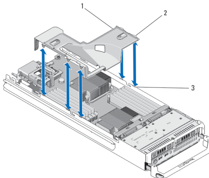
図 6. 冷却用エアフローカバーの取り外しと取り付け
