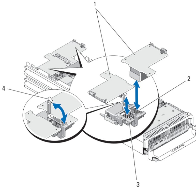
図9. メザニンカードの取り外しと取り付け
